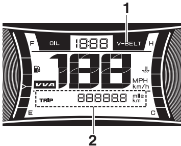
1. 三角皮带更换指示器“V-BELT” 2. 三角皮带更换行程表
